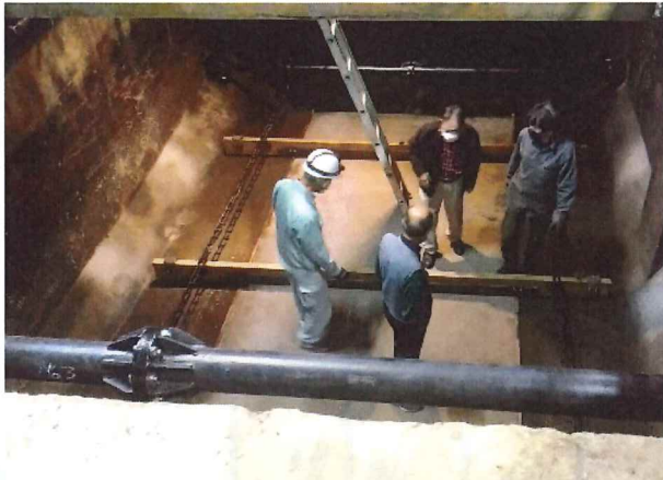
沈殿槽内で劣化部品交換の確認
